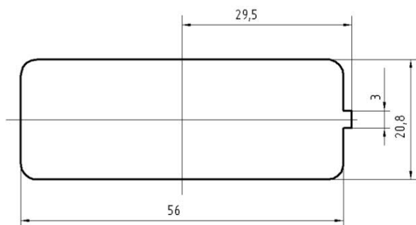
Рис. 1. Размеры места установки переключателя стеклоподъемника 11180-3709613-10
