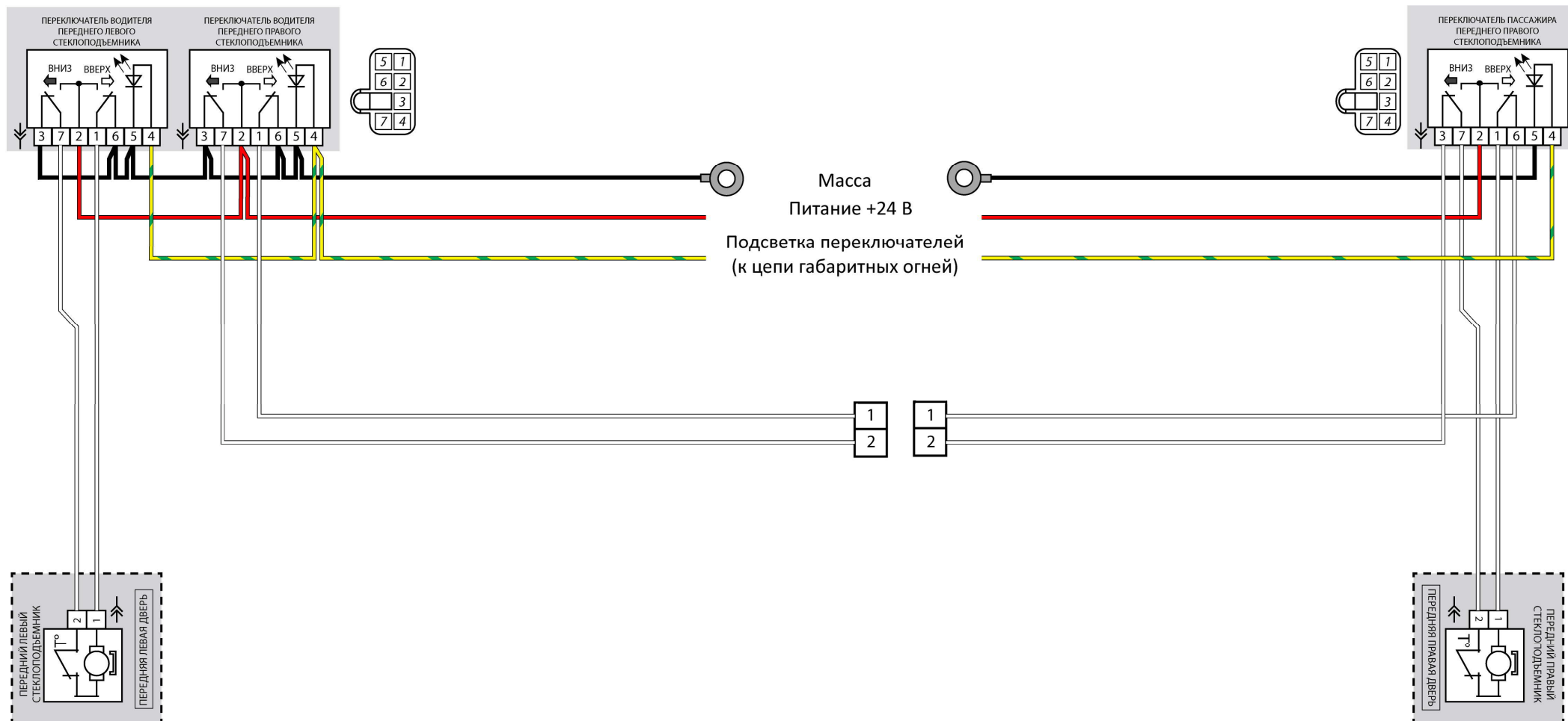
Рис. 2. Схема подключения электропроводки стеклоподъемников
