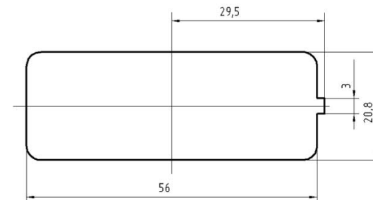
Рис. 1. Размеры мест для установки переключателя стеклоподъемника 921.3709-02.
